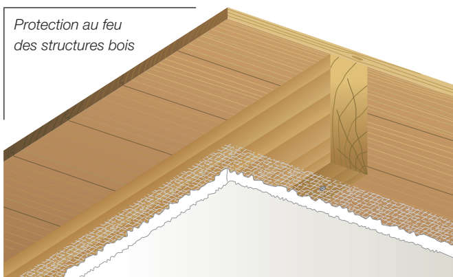
Protection au feu des membranes horizontales
