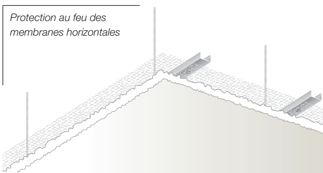
Protection au feu des planchers mixtes
